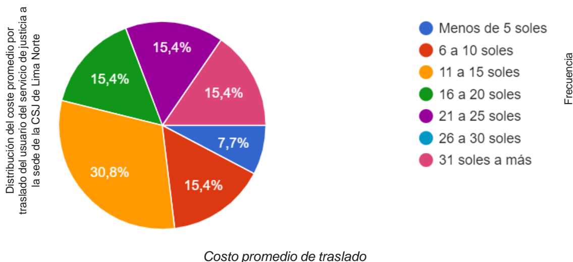
Figura n.º 13 Costes promedio de traslado del usuario del servicio de justicia a la CSJ de Lima Norte
